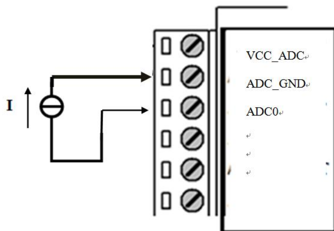
4-20mA 模拟量输入接线示意图：
